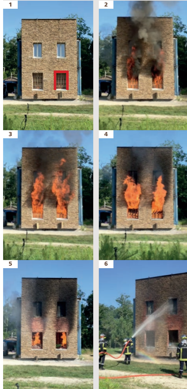
Das garantierte murogeopietra Verfahren auf EPS bewahrt die Festigkeit der Fassade.
